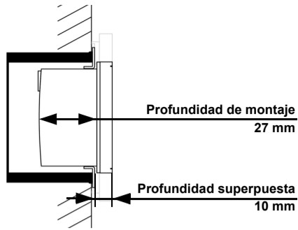
Fig. 1: Dibujo de sección. El Pulsador Cala KNX M-T se ajusta a una caja de dispositivos estándar (Ø 60 mm, profundidad 42 mm). ¡El marco no está incluido en el volumen de suministro!
