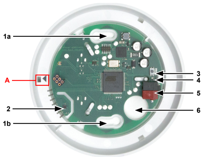
Fig. 2 1 a+b Ranuras para sujeción (espacio entre orificios 60 mm) 2 Sensores de temperatura, humedad 3 Teclado programador 4 LED de programación 5 Borne KNX Bus +/- 6 Entrada para cable A Marca para alinear la tapa
