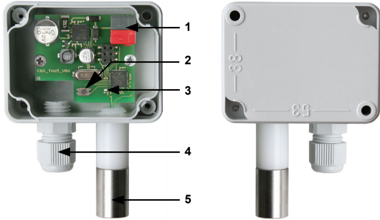
Fig. 1 Gabinete abierto, placa de cir- cuitos
