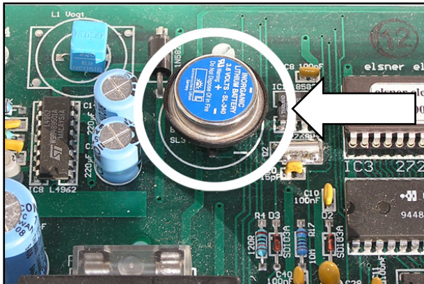
Abb. 1: Knopfbatterie SL 340 in der Steuerung WS100
