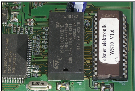
Abb. 3: S-Ram-Batterie in der Steuerung WS10
