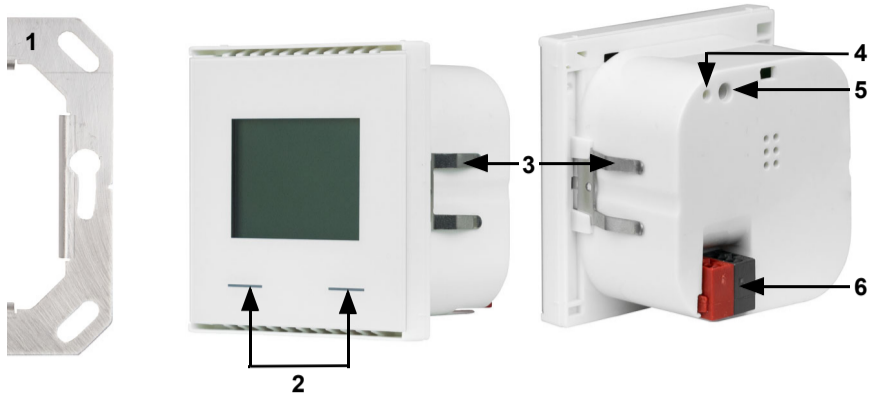
Abb. 2 1 Tragrahmen 2 Touch-Tasten 3 Rasten 4 Programmier-LED (versenkt) 5 Programmier-Taste (versenkt) zum Einlernen des Geräts 6 KNX-Klemme BUS +/-
