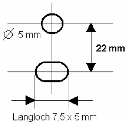
Abb. 7 a: Bohrplan
