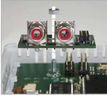
Abb. 2 Schrauben Sie die Schnittstelle fest, wie in der Detailsicht (links) zu sehen.
